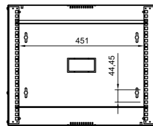
B-B KESİT GÖRÜNÜŞ
